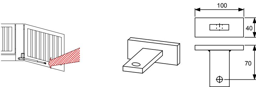
Bild 7 Anbauteil Torflügel
